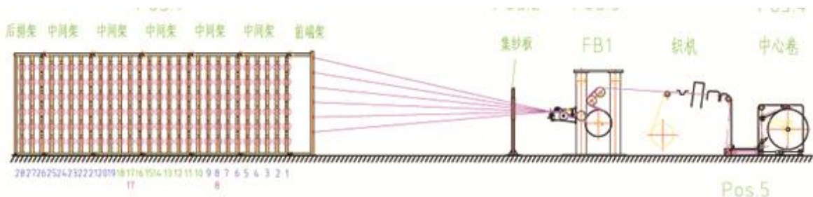
我们可提供的完整碳布织造生产线示意图
